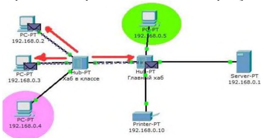
Рис.1.11. Прохождение пакета. Второй этап Если пакеты каким-то узлам не предназначены, они просто игнорируют их (рис.1.12). Когда пакет вернётся обратно, мы увидим подтверждение соединения.
