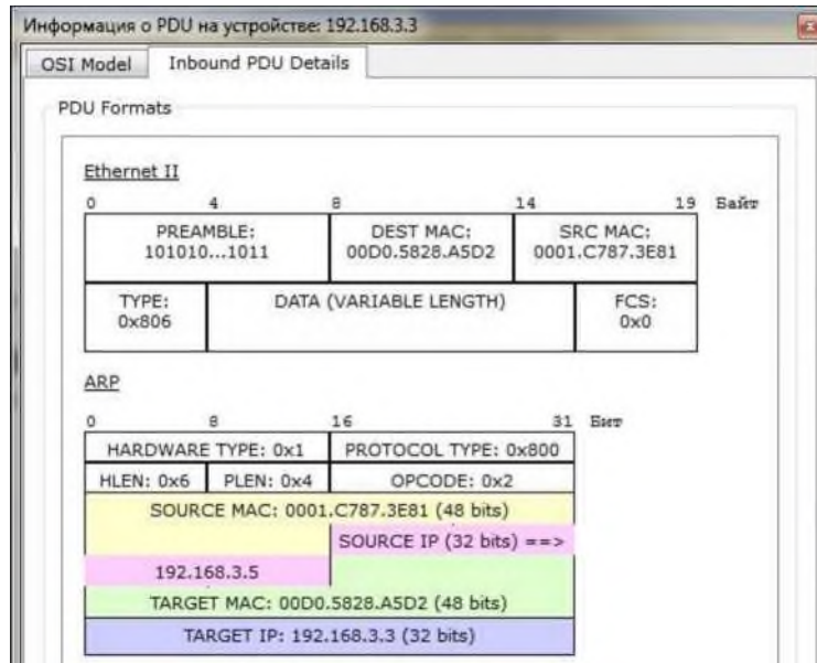
Рис. 2.14. Формат пакета ARP-ответа
