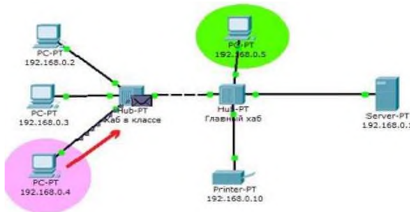
Рис.1.10. Прохождение пакета. Первый этап Концентратор по определению повторяет пакет на всех остальных портах (рис.1.11)
