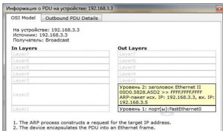
Рис. 2.13. Формат пакета ARP-запроса
